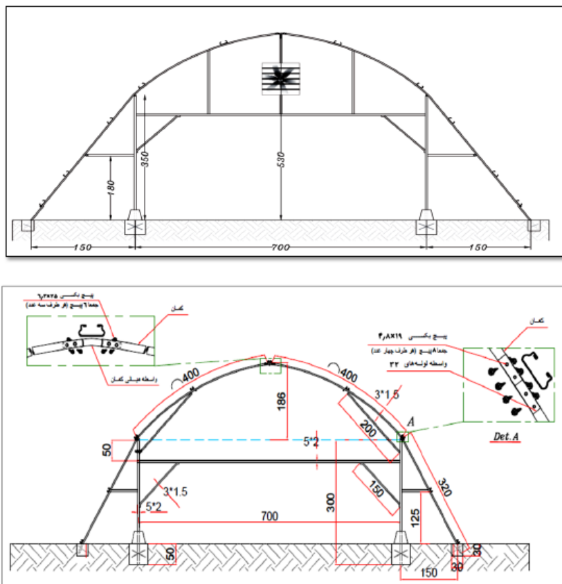
شکل ۱۱. مشخصات ظاهری و سازه گلخانه تیپ تونلی تک دهانه با دیواره باد شکن
