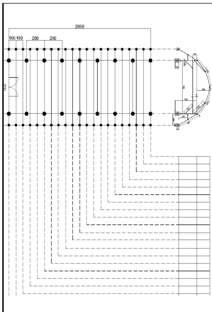
شکل ۱۲. پلان سه نمای گلخانه تیپ تونلی تک دهانه، با دیواره باد شکن
