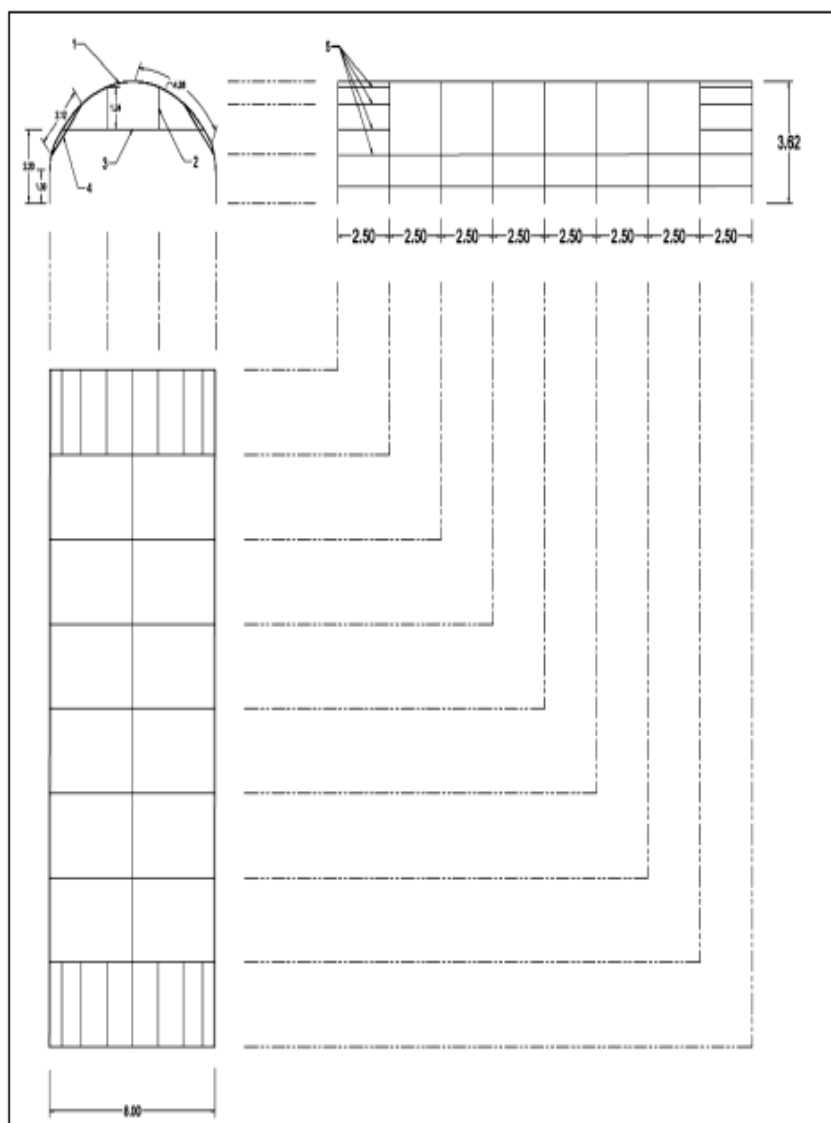
شکل ۱۶. پلان سه نمای گلخانه تونلی ایستاده
