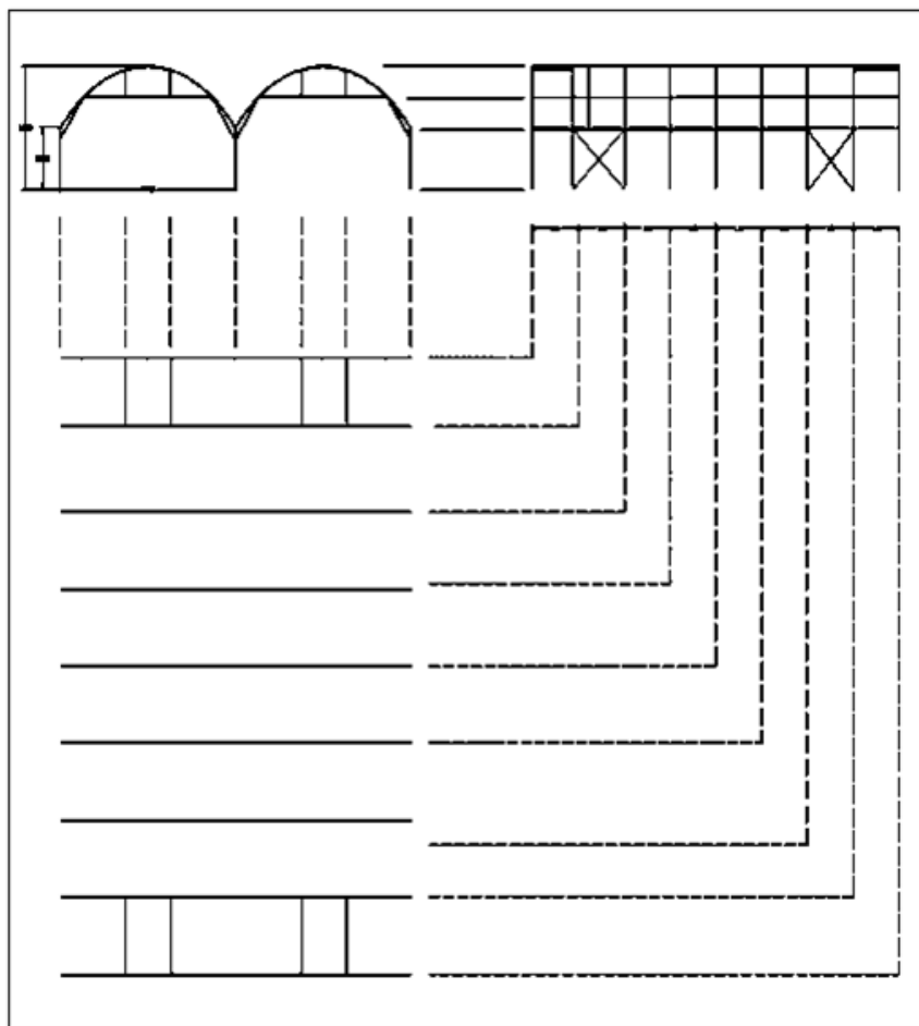
شکل ۲۷. پلان سه نمای گلخانه تونلی تیپ دو دهانه ایستاده
