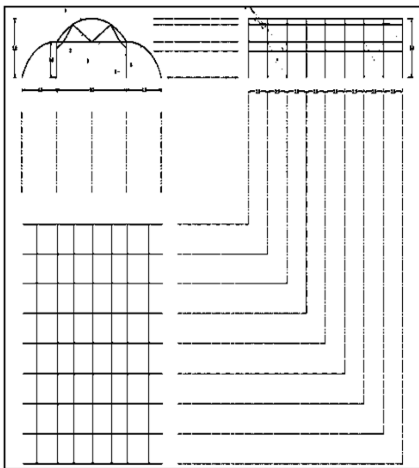
شکل ۲۱. پلان سه نمای گلخانه تونلی بلند دو طرف باد شکن
