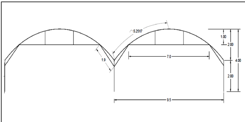
شکل ۲۵. ساین پیشنهادی گلخانه تونلی دو دهانه
