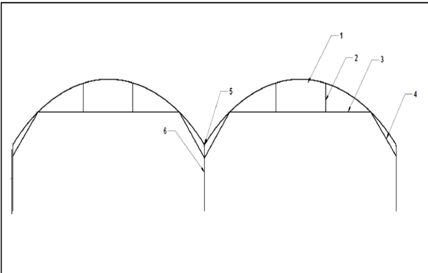
شکل ۲۶. ساین پیشنهادی گلخانه تونلی دو دهانه
