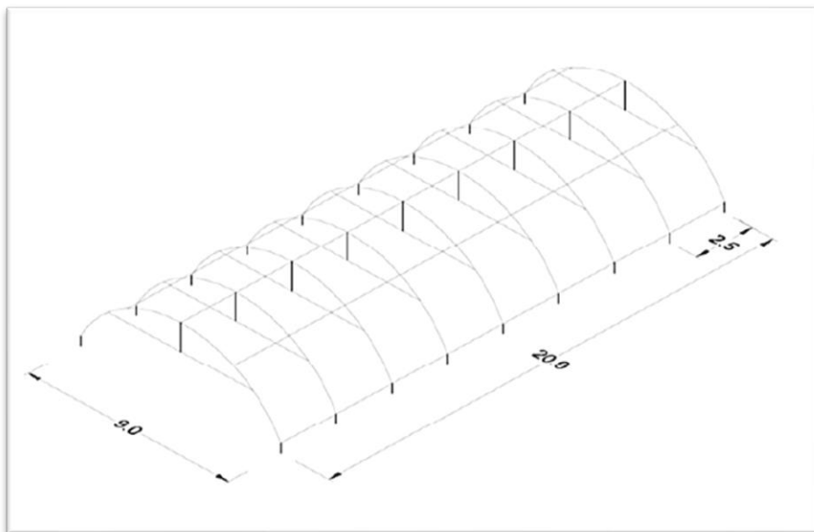
شکل ۹. طرح تیپ پیشنهادی برای گلخانه کوچک مقیاس تونلی ساده یا کوانست Quons
