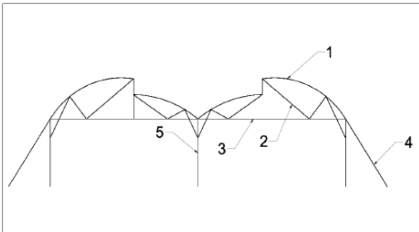
شکل ۳۰. سایز و مشخصات المان‌های سازه گلخانه تونلی دو دهانه تیپ دندانه‌ای
