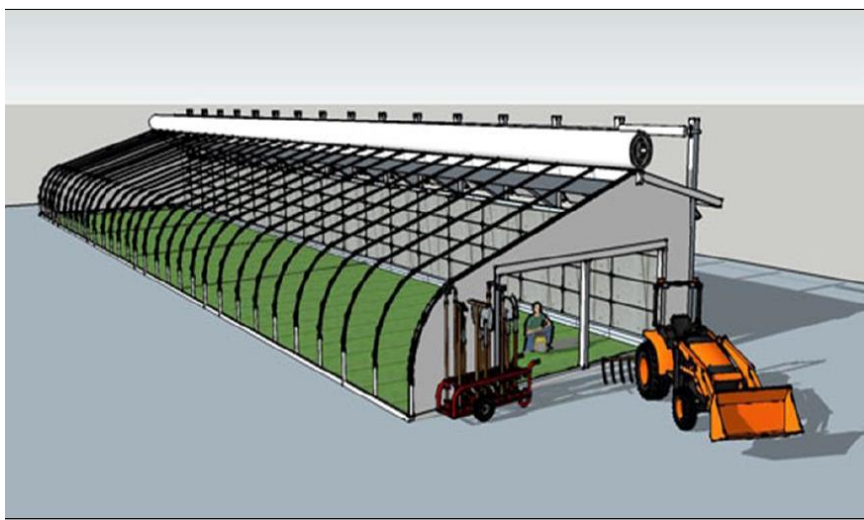
شکل ۳۱. شکل ظاهری گلخانه یک طرفه طرح خورشیدی
