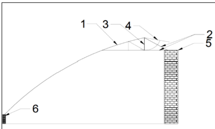
شکل ۳۲. سایز و اندازه گلخانه یک طرفه طرح خورشیدی
